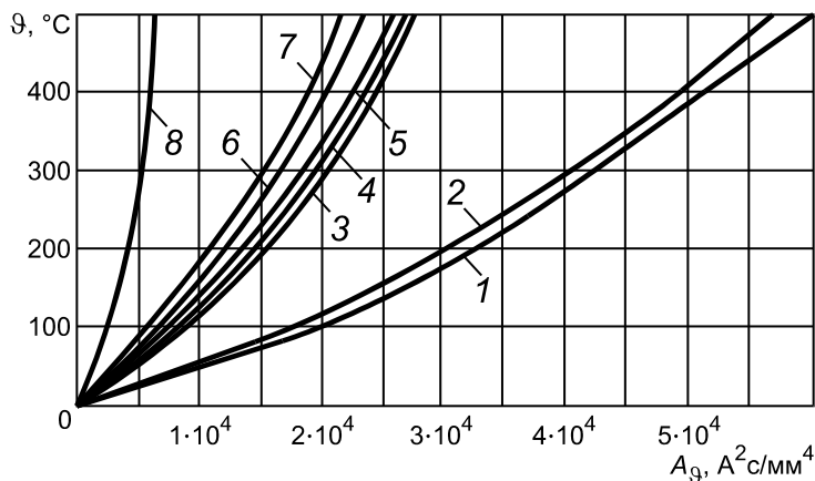
Материалы проводников: 1 — ММ; 2 — МТ; 3 — АМ; 4 — АТ; 5 — АДО, АСТ; 6 — АД31Т1; 7 — АД31Т; 8 — Ст3
