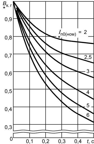
Рисунок 10 — Кривые для определения V_{*к.г} от синхронных генераторов с тиристорной системой самовозбуждения
