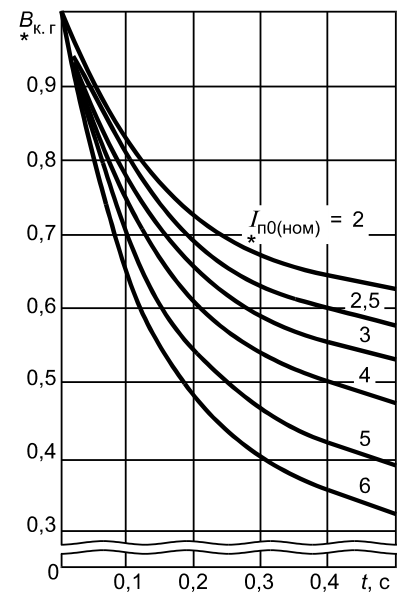
Рисунок 11 — Кривые для определения V_{*к.г} от синхронных генераторов с диодной бесщеточной системой самовозбуждения
