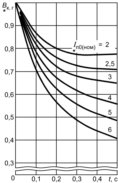
Рисунок 9 — Кривые для определения V_{*к.г} от синхронных генераторов с тиристорной независимой системой возбуждения
