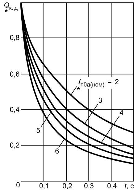
Рисунок 18 — Кривые для определения Q_{*к.д} от асинхронного электродвигателя
