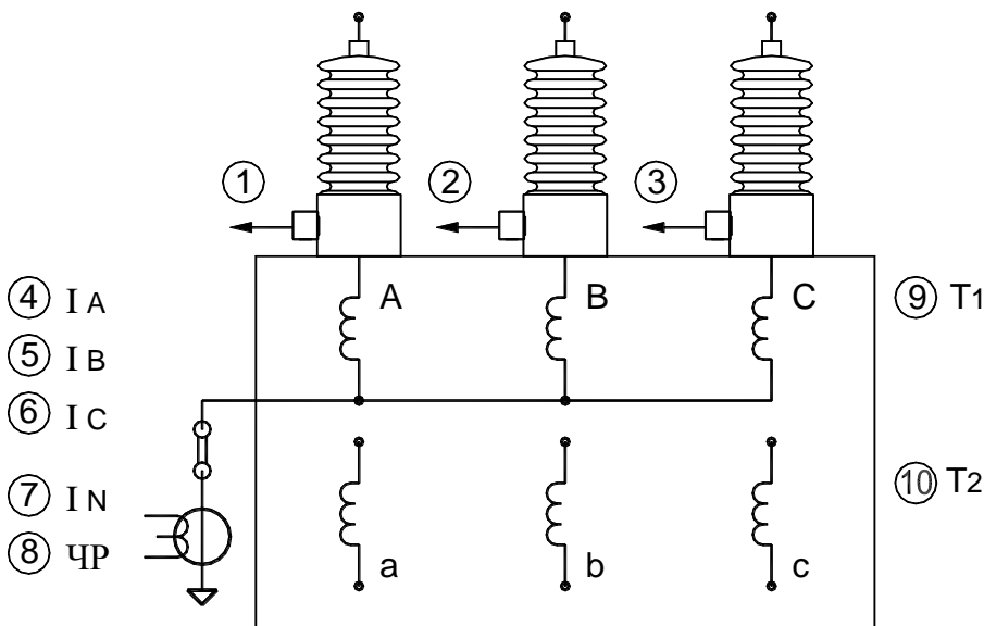
Рисунок 1.1 Места установки датчиков системы
